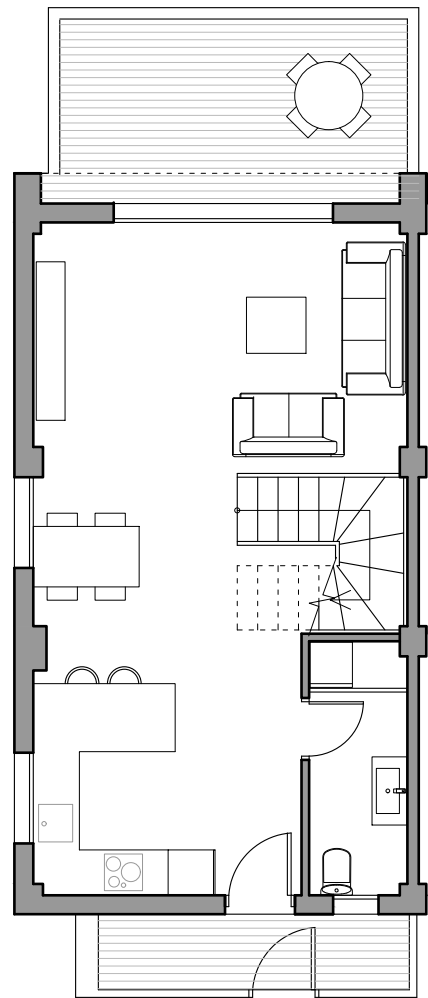
PLANTA BAJA
